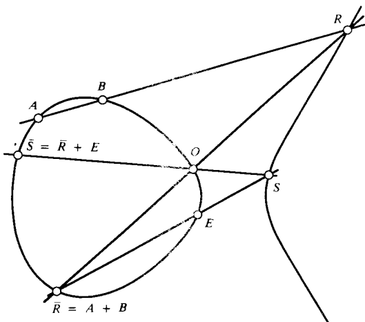
Кубическая кривая и групповой закон на ней
