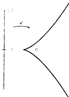
Полукубическая парабола y^2 = x^3
