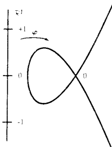
Декартов лист y^2 = x^3 + x^2
