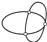
2P_1 + P_2 + P_3
